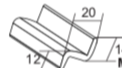
Perfil Z
